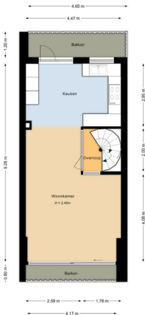
Eerste verdieping Maarten Kruytstraat 6 Noordwijk
